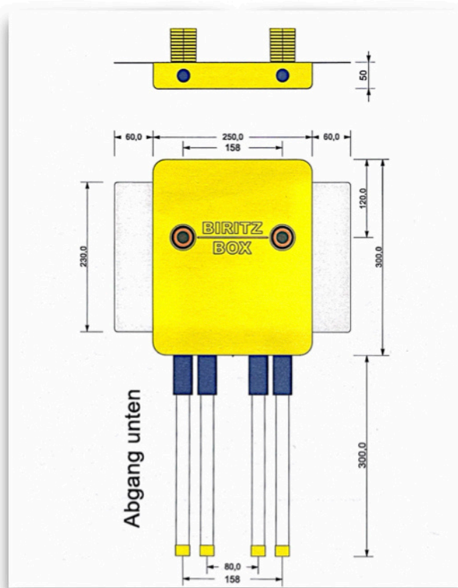
Montage Box für Dusche und Badewanne durchgeschliffen mit Bauhülse Mauerwerk - Trockenbau
