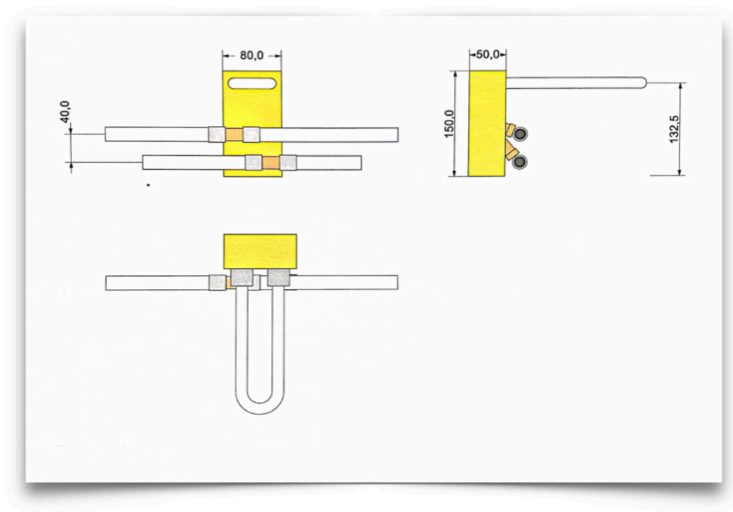
Montage Box für Heizkörper Aufputzsockelbox - Mauerwerk
