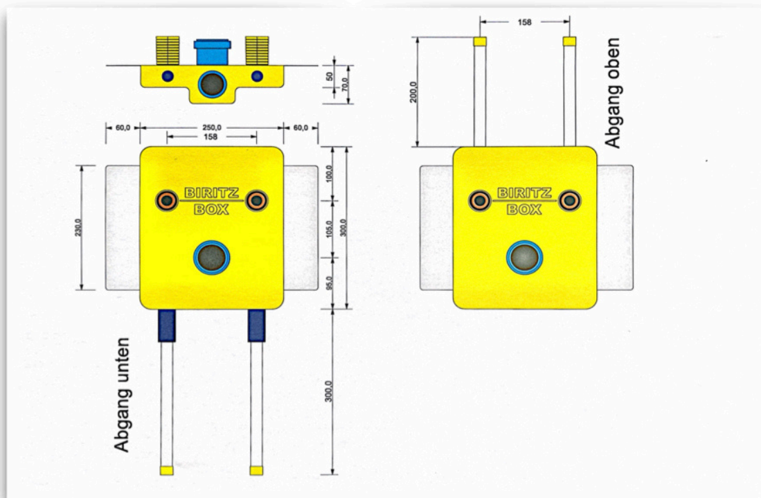
Montage Box für Spüle mit Bauhülse - Trockenbau
