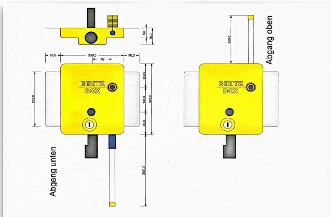
Montage Box für Waschmaschine mit Bauhülse - Trockenbau
