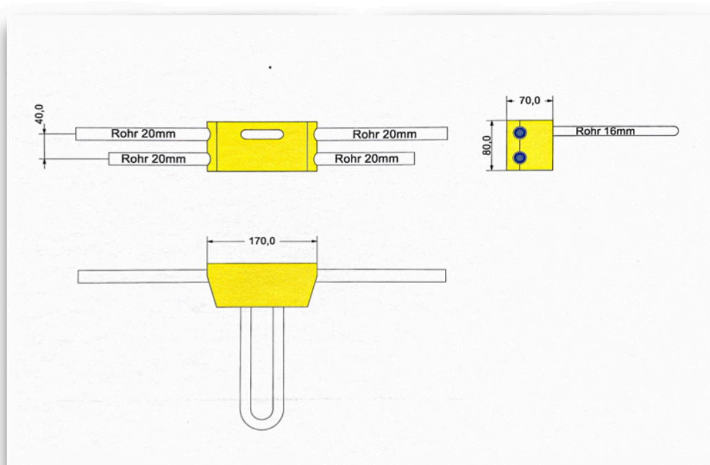
Montage Box für Heizkörper Sockelbox - Mauerwerk
