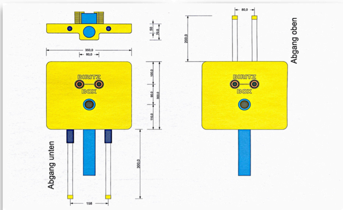
Montage Box für Waschtisch/Handwaschbecken mit Bauhülse - Mauerwerk
