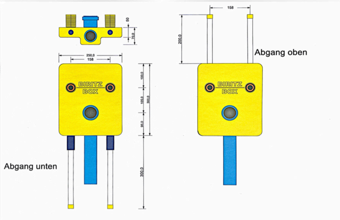
Montage Box für Spüle mit Bauhülse - Mauerwerk
