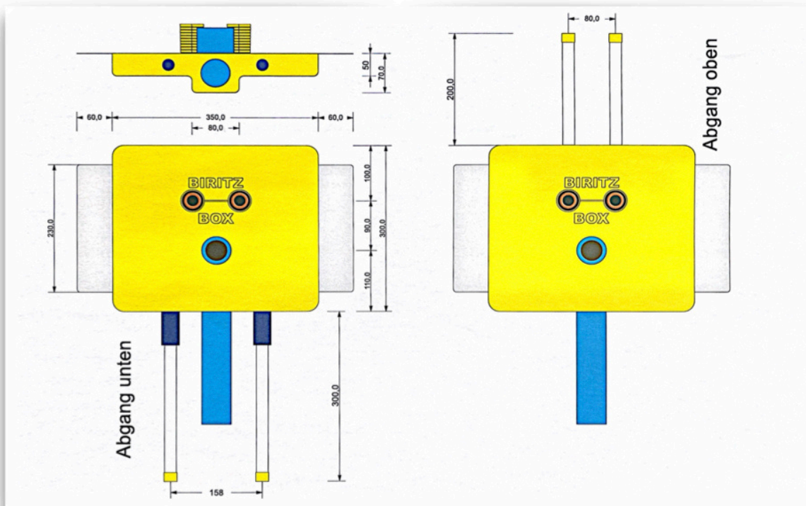
Montage Box für Waschtisch/Handwaschbecken mit Bauhülse - Trockenbau
