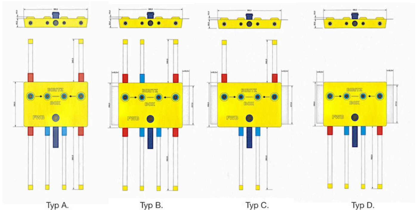
Montage Box für Fernwärmebox - Mauerwerk und Trockenbau
