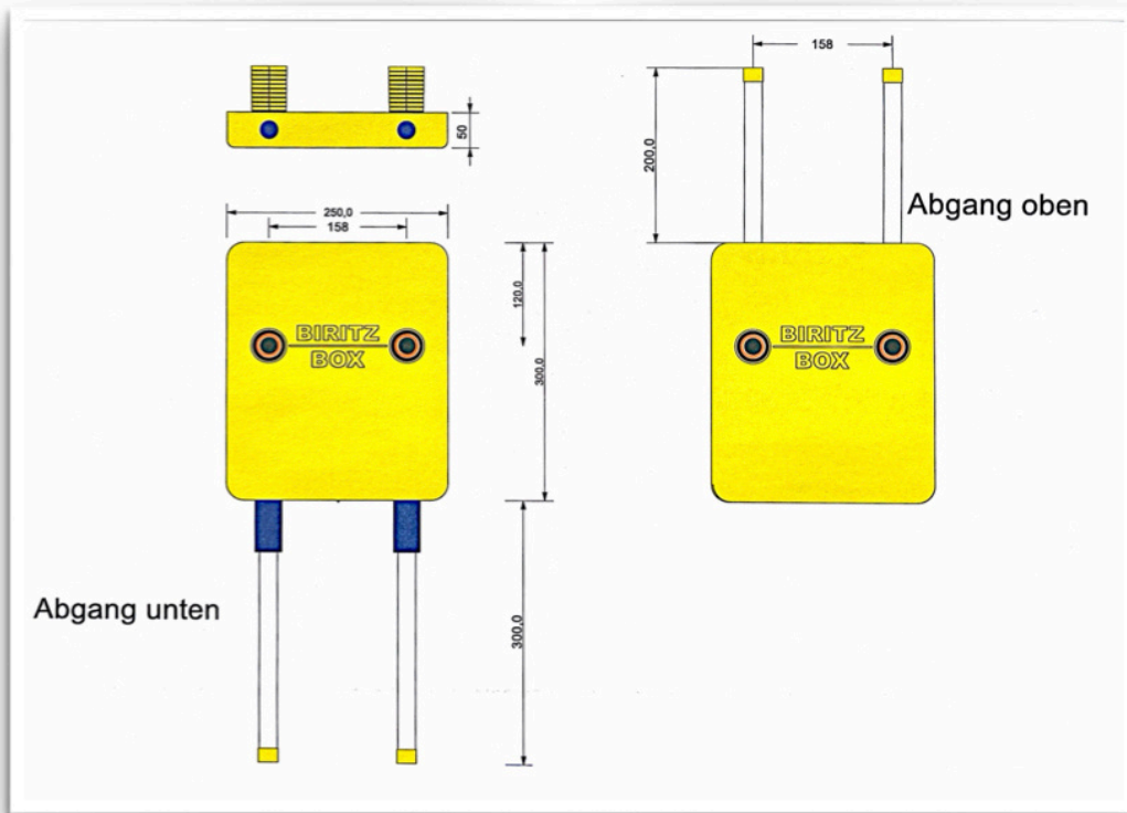
Montage Box für Dusche und Badewanne mit Bauhülse - Mauerwerk
