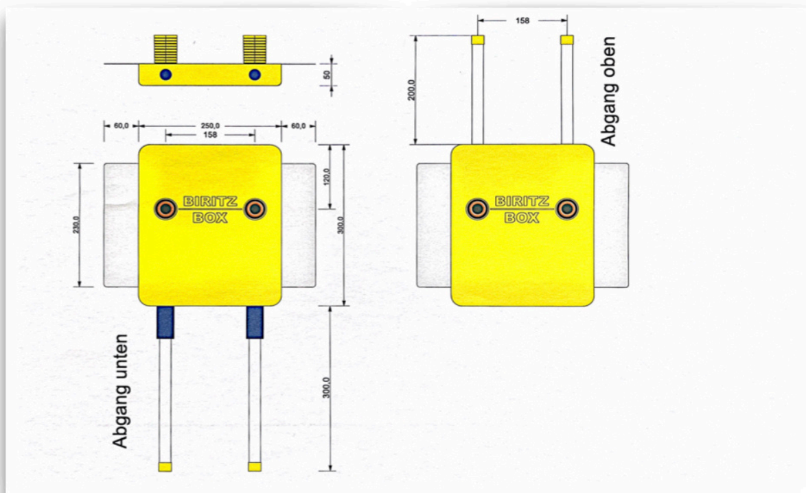
Montage Box für Dusche und Badewanne mit Bauhülse - Trockenbau
