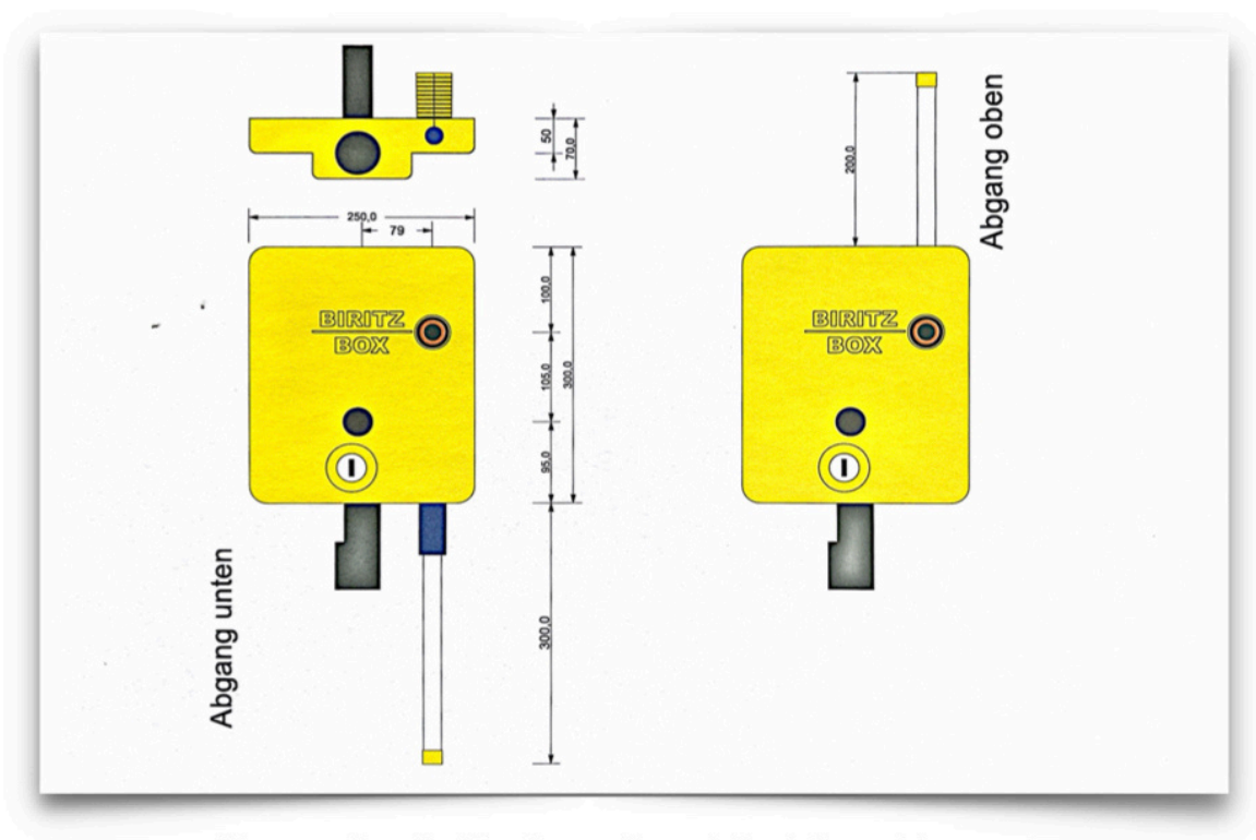
Montage Box für Waschmaschine mit Bauhülse - Mauerwerk
