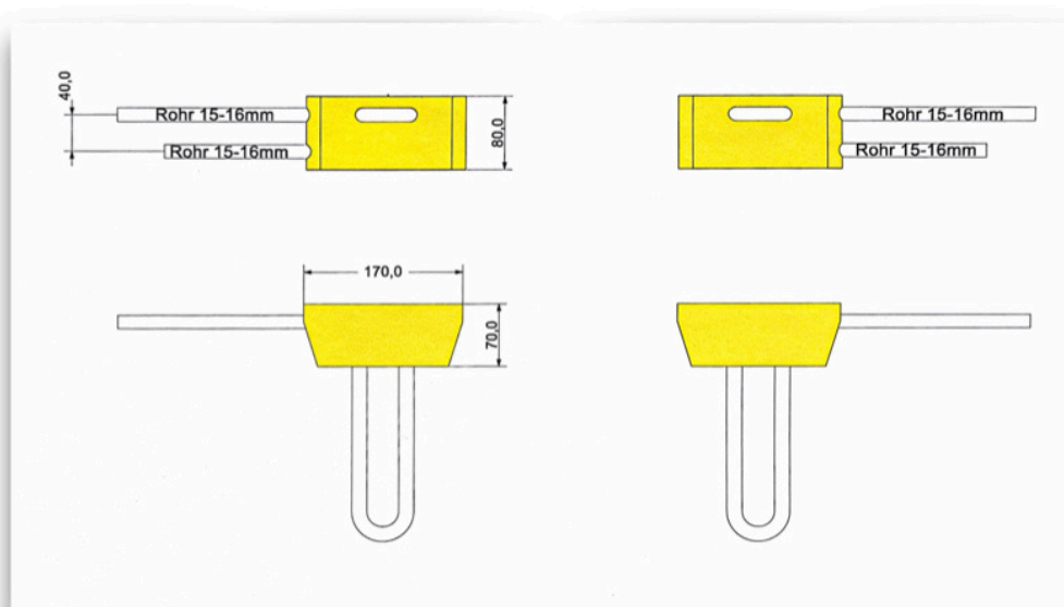
Montage Box für Heizkörper Sockelbox Links und Rechts - Mauerwerk
